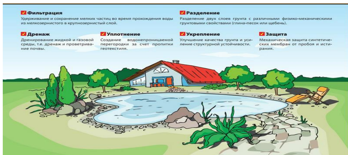
Рис.1. Основные функции строительного геотекстиля
